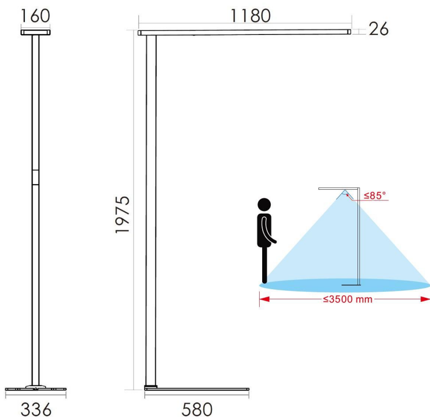
Integrierte Sensoreinheit
